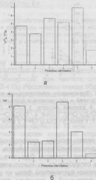
Рис. 1. Зависимость среднего значения микротвердости (а) и коэффициента износостойкости (б) в поверхностном слое от режима наплавки: 1 – \text{Cr}_3\text{C}_2 ; 2 – \text{Cr}_3\text{C}_2/\text{Cr}=1 , 1 слой; 3 – \text{Cr}_3\text{C}_2/\text{Cr}=1 , 2 слоя; 4 – \text{Cr}_3\text{C}_2/\text{Cr}=2 , 1 слой; 5 – \text{Cr}_3\text{C}_2/\text{Cr}=2 , 2 слоя; 6 – сталь Ст3
