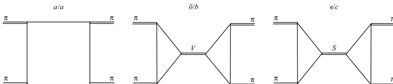
Рис. 4. Диаграммы, определяющие амплитуду \pi\pi -рассеяния
