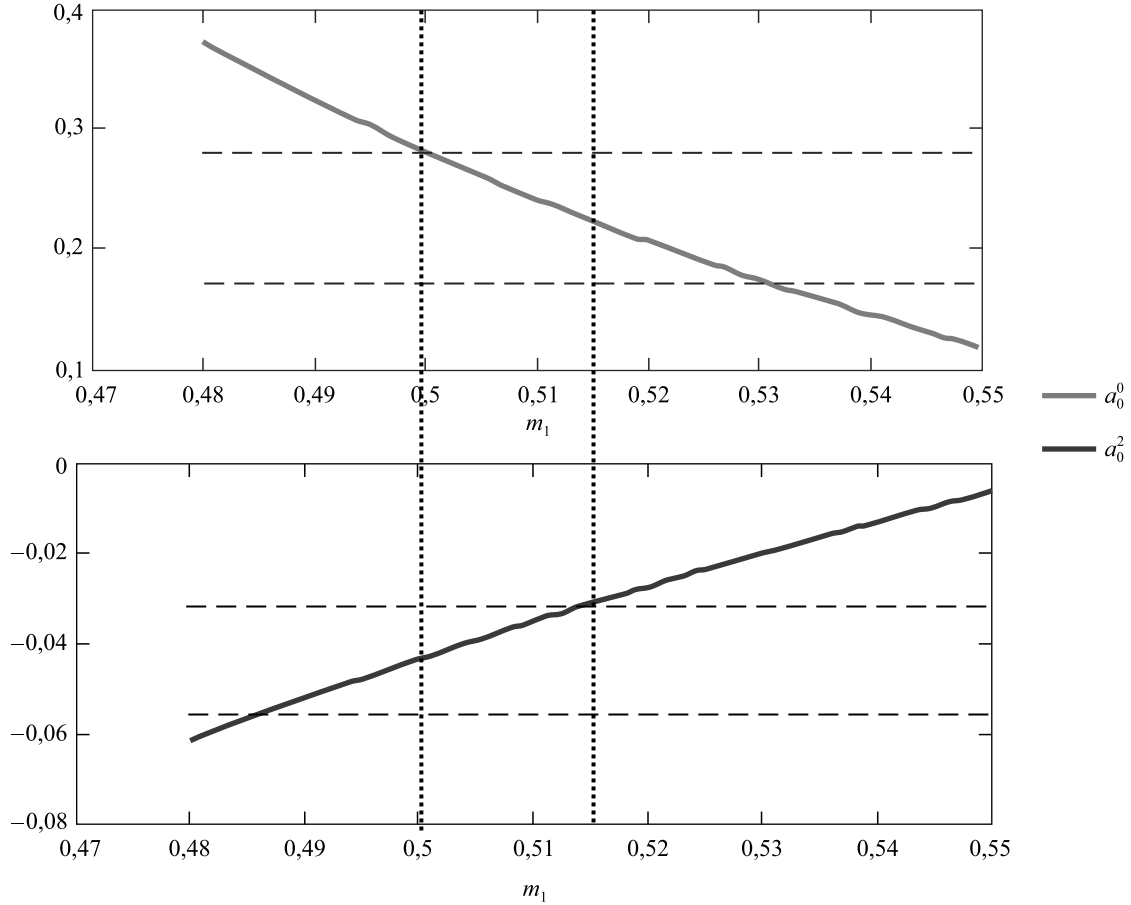
Рис. 5. Зависимости численных значений длин \pi\pi -рассеяния a_0^0 и a_0^2 от массы m_1 мезона f_0(600) .
