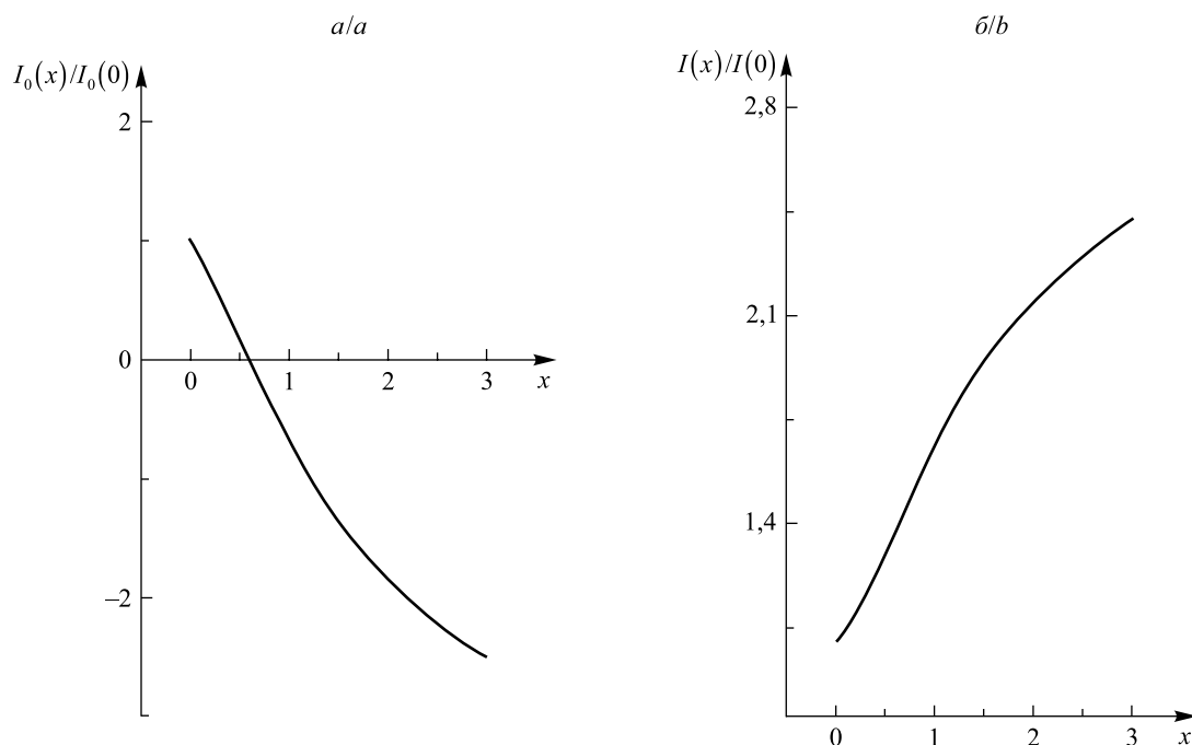
Рис. 3. Зависимость структурных интегралов, определяющих матричный элемент распада S \rightarrow PP , от массы скалярного мезона
