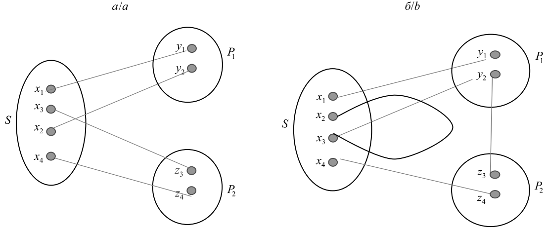
Рис. 8. Кварковые диаграммы, описывающие распад S \rightarrow PP в четырехкварковой схеме
