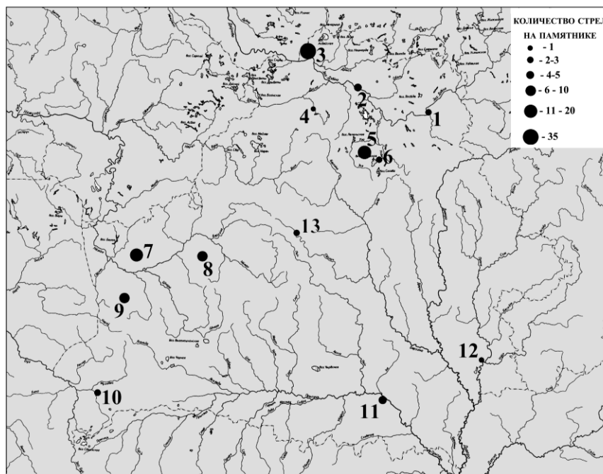
Мал. 5. Распаўсюджанне ланцэтападобных стрэл на тэрыторыі Беларусі
