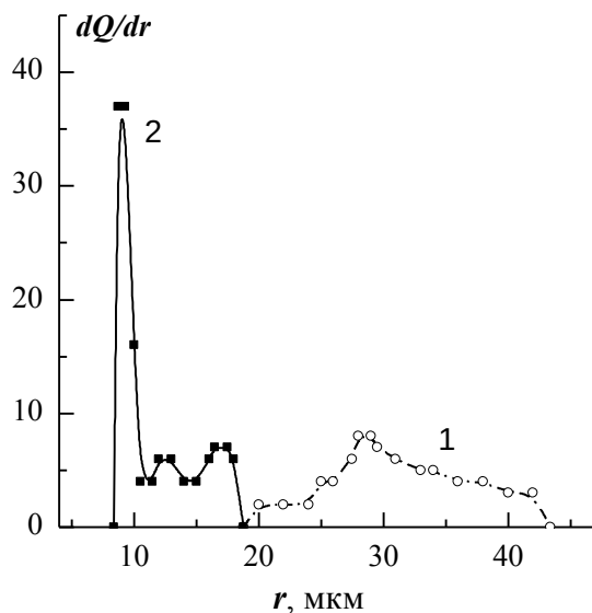
Рис. 2. Дифференциальные кривые распределения по размерам частиц суспензий образцов ОУ-А: 1 – исходного; 2 – модифицированного
