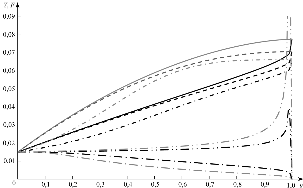
Кривые доходности (черные) и форвардные кривые (серые) для моделей: № 1 – сплошные; № 2 – пунктир; № 3 – штрихпунктир; № 4 – длинный штрихпунктир; № 5 – двойной штрихпунктир Yield curve (black) – and forward rate curve (gray), model: No. 1 – solid; No. 2 – dotted line; No. 3 – dash-dotted; No. 4 – long dash-dotted; No. 5 – double dash-dotted
