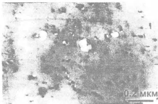
Рис.1. Гелиевые поры в ферритном зерне углеродистой стали (Fe+0,58%C): а - общий вид, б - поры, заполненные углеродом.
