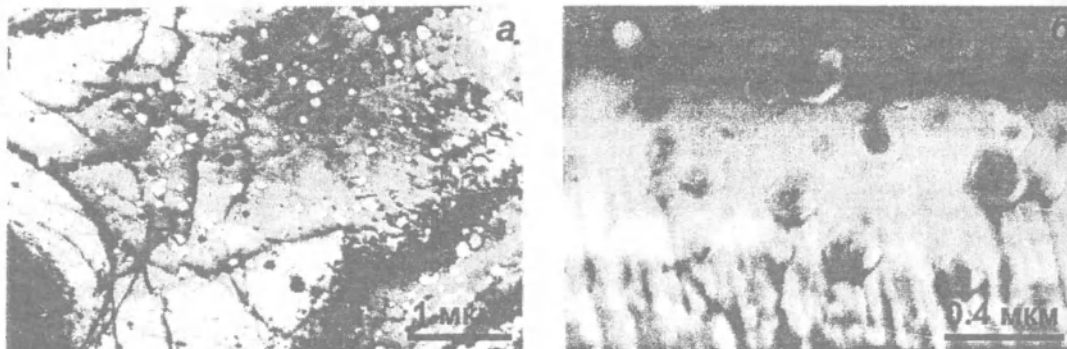
Рис.1. Гелиевые поры в ферритном зерне углеродистой стали (Fe+0,58%C): а - общий вид, б - поры, заполненные углеродом.
