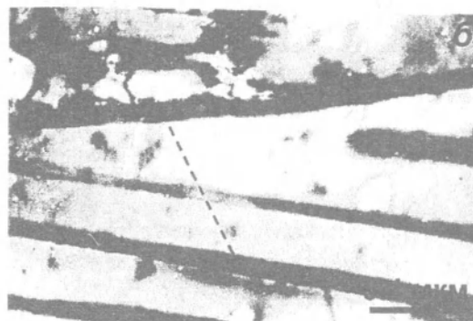
Рис.4. Развитие полосчатой (пунктирная линия) структуры распределения гелиевых пор в ферритном (а) и перлитном (б) зернах.
