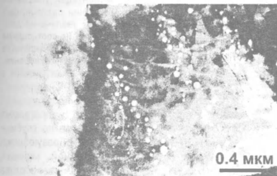
Рис.4. Развитие полосчатой (пунктирная линия) структуры распределения гелиевых пор в ферритном (а) и перлитном (б) зернах.
