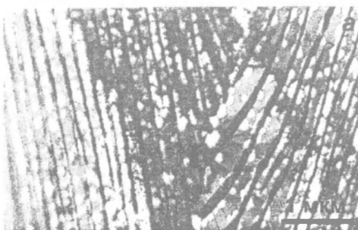
Рис.3. Гелиевые поры в перлитном зерне углеродистой стали (Fe+0,58%C): а - общий вид, б - гелиевые поры на цементитных пластинках.
