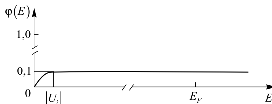
Рис. 2. Горизонтальная линия примерно воспроизводит ход функции \varphi(E) = \left[ \ln^2 \left( \frac{E}{|U_i|} \right) + \pi^2 \right]^{-1}
