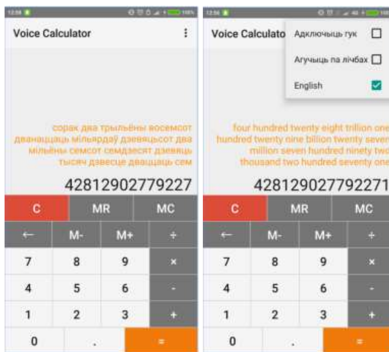
Мал. 1. Галоўны экран, функцыі і вывад вынікаў у праграме «Гаворачы калькулятар»
