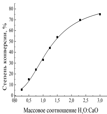
Рис. Зависимость степени конверсии от: а – массового соотношения H_2O : CaO и б – температуры термообработки
