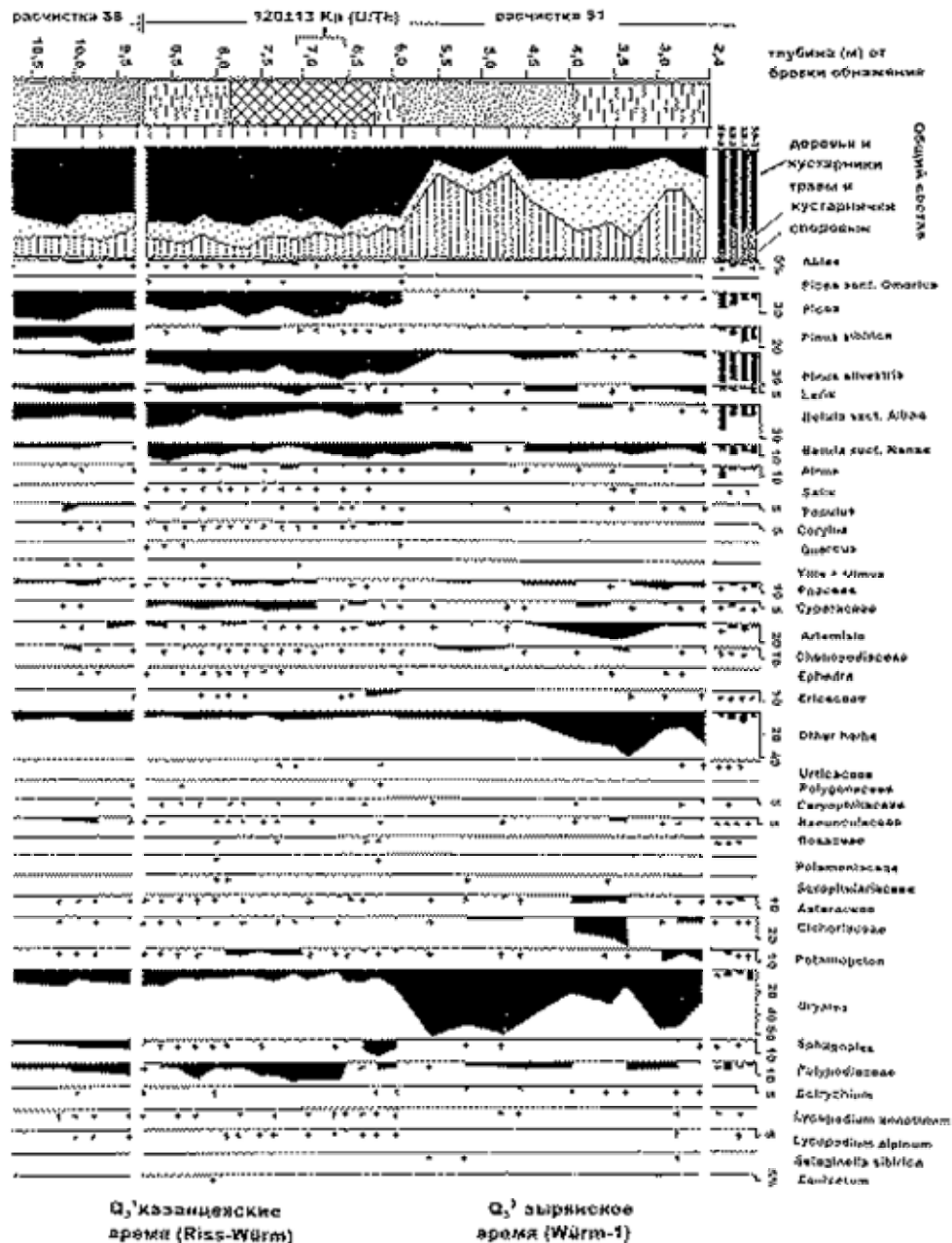
Рис. 5. Спорово-пыльцевая диаграмма разреза Бедоба. Крестиком показано количество менее 2%; ss — поверхностные пробы. Остальные обозначения см. на рис. 2 и 3
