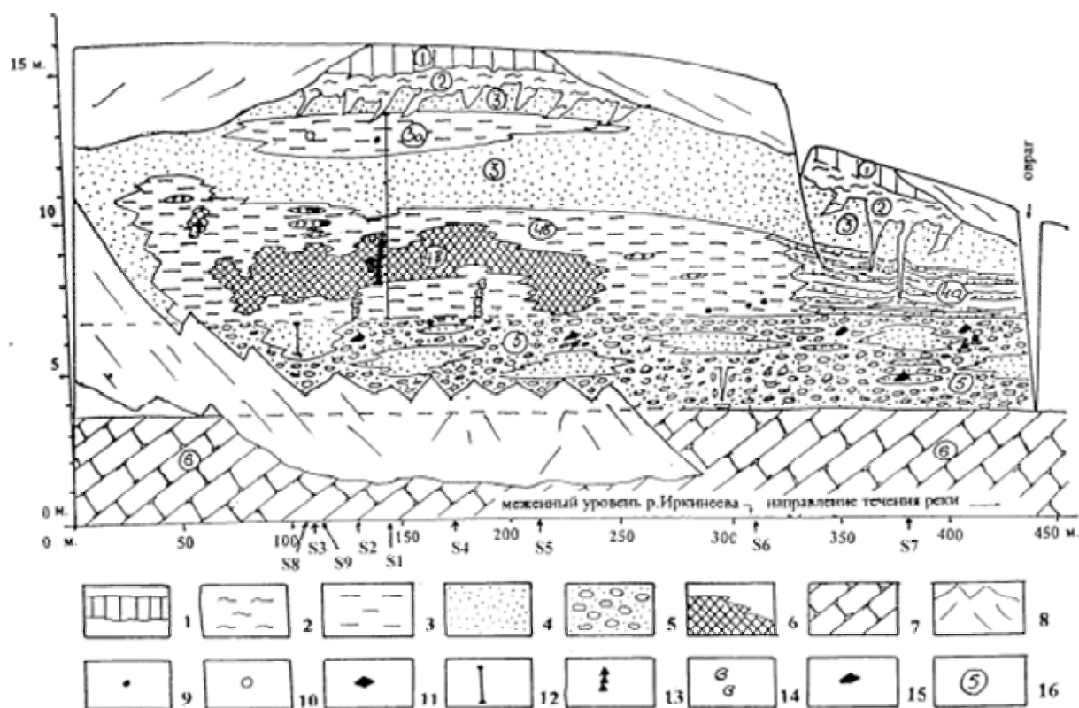
Рис. 2. Обобщенная схема строения разреза Бедоба. S1–9 расположение основных расчисток: 1 — суглинок серый, лессовидный; 2 — суглинок и глина вишнево-коричневая; 3 — глина сизо-серая дочерной; 4 — песок; 5 — галечник ожелезненный до железистого конгломерата; 6 — торф; 7 — алеврит палеозоя (цоколь террасы); 8 — наиболее мощные осыпи; 9 — положение ^{14}\text{C} -дат, полученных в 1960-е годы; 10 — положение ^{14}\text{C} -дат, полученных в 2003 г; 11 — положение уран-ториевой даты; 12 — интервалы разреза, по которым сделан спорово-пыльцевой анализ; 13 — места отбора образцов на карполопию (К1-7); 14 — места отбора образцов на малакофауну; 15 — положение раковин унионид; 16 — номера слоев: 1 и 2 — покровная толща, 3 — констративный аллювий (3а — глины фации вторичного водоема), 4 и 5 «нормальный» аллювий (4а — пойменные фации, 4б — глины и 4в — торфяник старичных фаций, 5 — русловые фации), 6 — цоколь террасы
