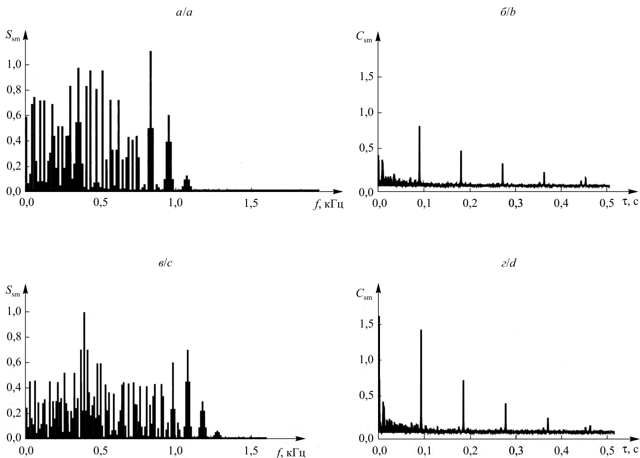
Рис. 3. Спектры (а, в) и кепстры мощности (б, г) при различных амплитудах микроколебаний \bar{x}_0 : 1,4 (а, б); 2,0 (в, г). Частоты: f_1 = 49 Гц; f_2 = 11 Гц. Глубина модуляции d = 0,5
