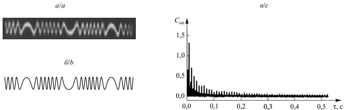
Рис. 1. Временной характер (а, б) и кепстр мощности (в) отклика лазера на гармонические колебания внешнего объекта с частотой 55 Гц: а – эксперимент; б, в – теория
