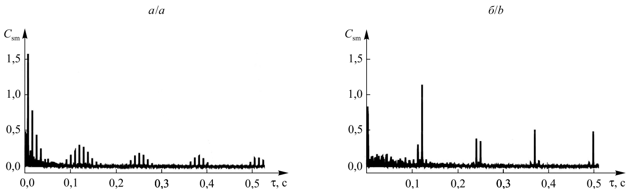
Рис. 2. Кепстры мощности сигнала самосмешения при амплитудной модуляции микроколебаний ( f_1 = 55 Гц) низкочастотным сигналом ( f_2 = 8 Гц).
