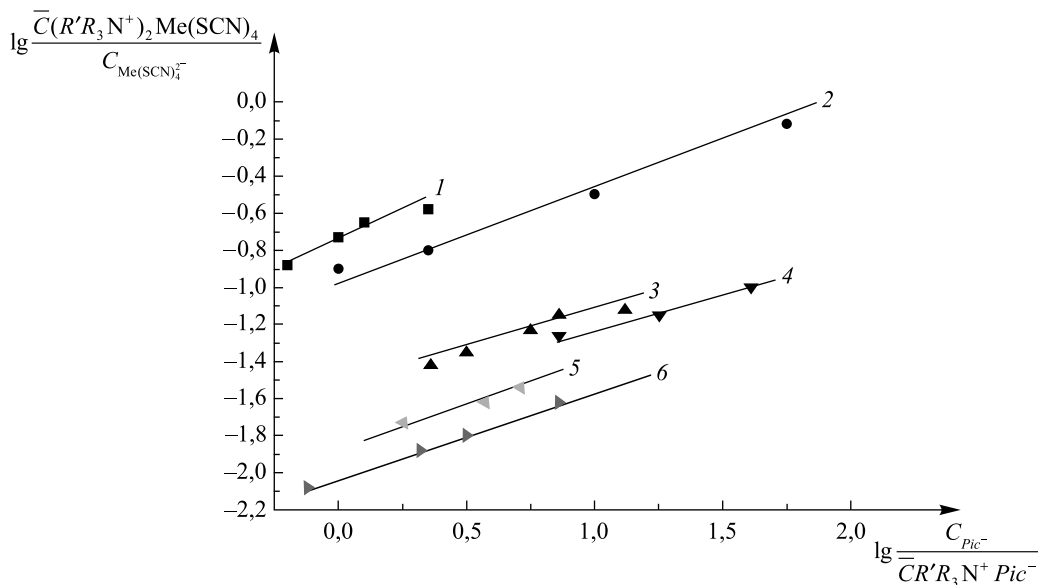
Рис. 2. Билогарифмическая зависимость коэффициента распределения металла от обратного коэффициента распределения пикрат-иона:
