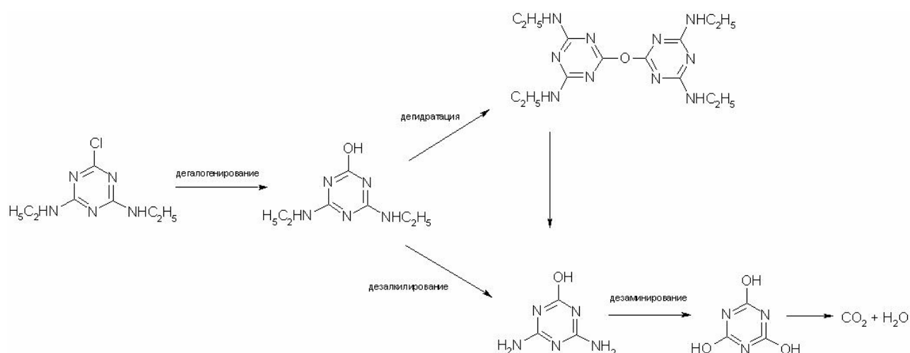
Рис. 1. Механизм деградации симазина ферментными системами штамма P. aurantica B-162.
