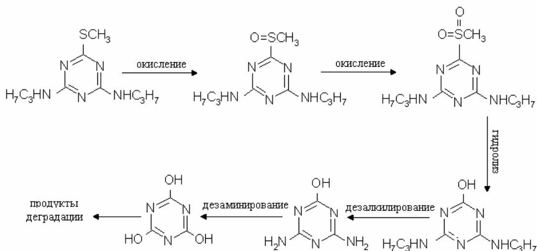
Рис. 2. Механизм деградации прометрина ферментными системами штамма P. aeruginosa B-7.
