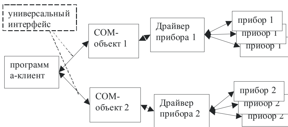
Рис 2. Трехуровневая структура многомодульного измерительного программного комплекса
