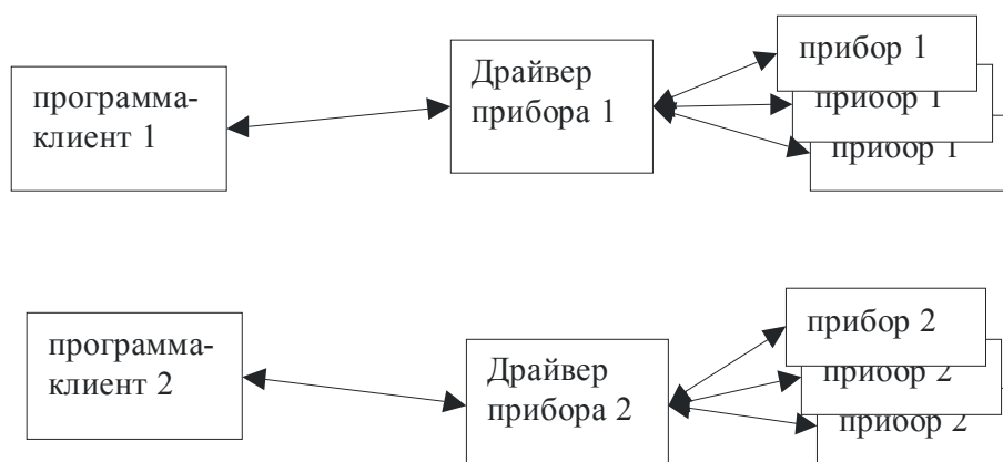
Рис 1. Двухуровневая структура многомодульного измерительного программного комплекса
