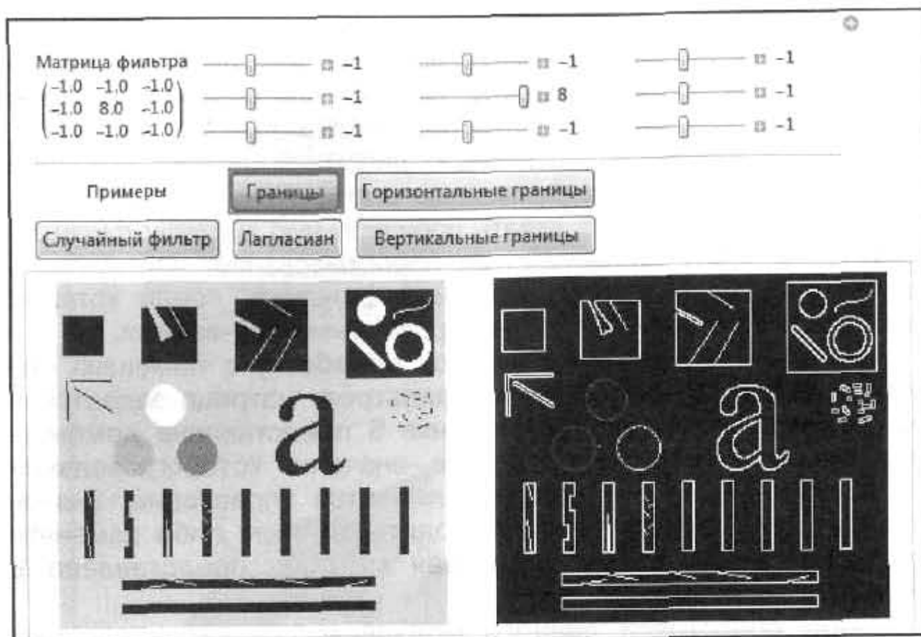
Рис. 4. Внешний вид панели управления и окна вывода модуля для демонстрации работы фильтра «Границы»
