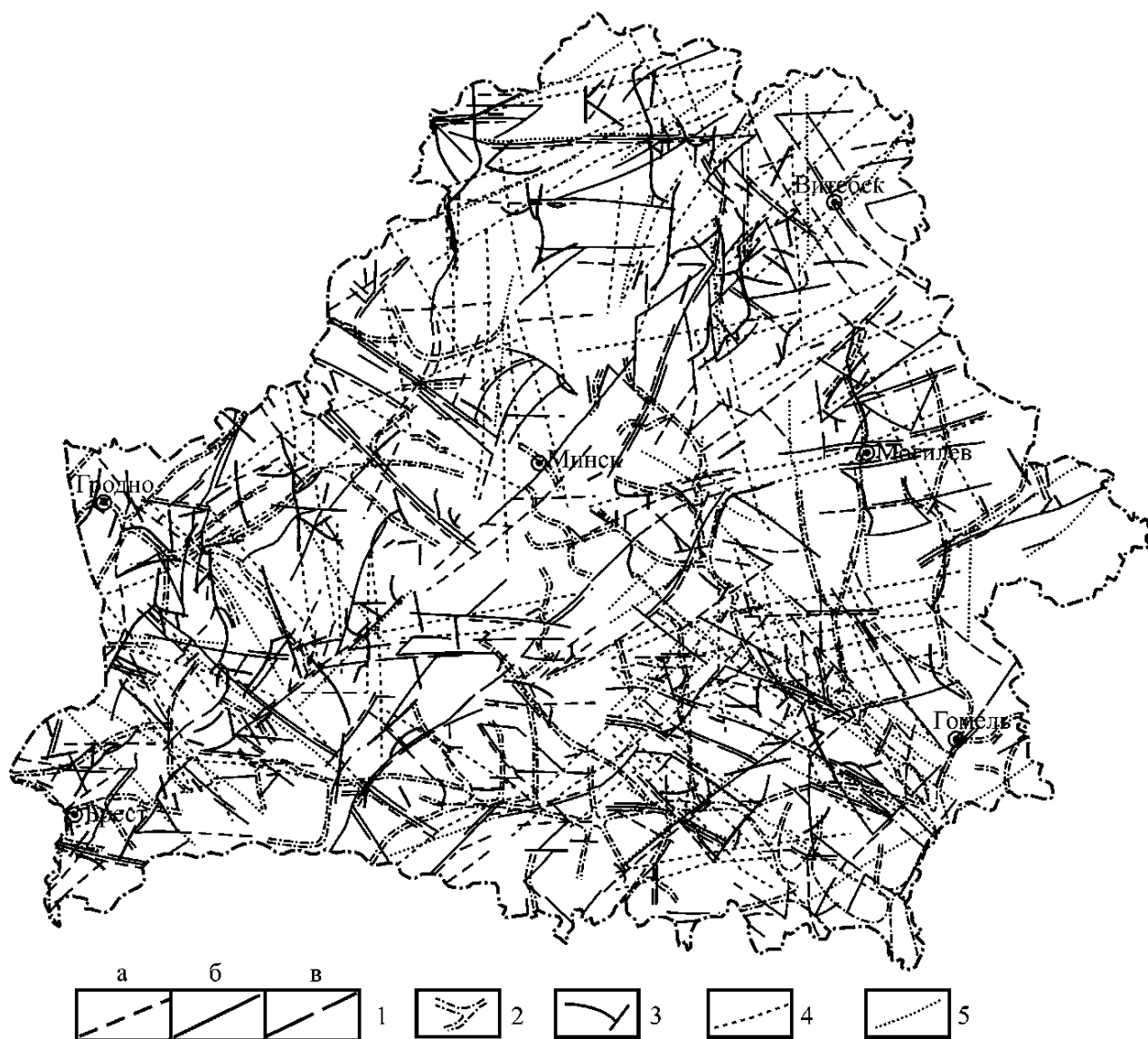
Рис. 1 – Геоактивные зоны на территории Беларуси: 1 – разрывные нарушения, проявившие активность в позднеплейстоцен-голоценовое (а), поздне-среднеплейстоценовое (б) и раннеплейстоценовое (в) время; 2 – погребенные речные долины; 3 – погребенные ледниковые ложбины; 4 – наиболее протяженные космолинеаменты; 5 – наиболее протяженные тополинеаменты
