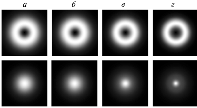
Рис. 1. Распределение интенсивности световых пучков на входе (а) и выходе (б–д) нелинейной среды. \alpha I_{01} = 1 (б), 5 (в), 30 (д).
