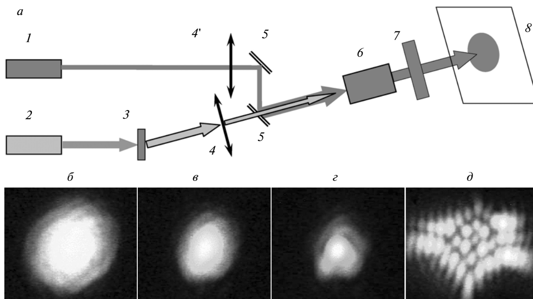
Рис. 3. Схема нелинейного взаимодействия световых пучков (а) (1 – гелий-неоновый лазер, 2 – лазер на иттрий-алюминиевом гранате, 3 – оптический транспарант, 4, 4' – линзы, 5 – зеркала, 6 – нелинейная среда, 7 – светофильтр, 8 – экран) и вид распределения интенсивности сигнального пучка на выходе из нелинейной среды в отсутствие пучка накачки (б) и при интенсивности накачки I = 40 (в) и 70 \text{ МВт} \cdot \text{см}^{-2} (г, д); фокусы сигнального пучка и пучка накачки разнесены на 2 см (б–г) либо совпадают (д).
