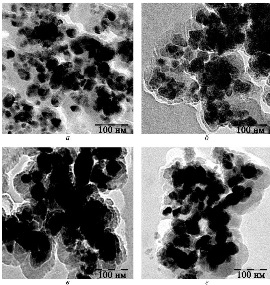
Рис. 1. ПЭМ-снимки частиц \text{SnO}_2 , синтезированных из \text{SnCl}_4 и \text{SnSO}_4 без и с использованием \text{NH}_3 \cdot \text{H}_2\text{O} в качестве стабилизаторов: а – из \text{SnCl}_4 (без стаб.) 700 °С; б – из \text{SnCl}_4 ( \text{NH}_3 \cdot \text{H}_2\text{O} ) 700 °С; в – из \text{SnSO}_4 (без стаб.) 600 °С; г – из \text{SnSO}_4 ( \text{NH}_3 \cdot \text{H}_2\text{O} ) 600 °С
