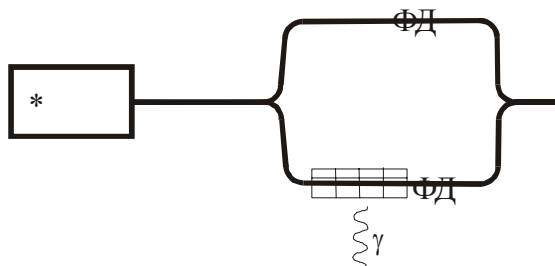
Рис. 1. Принципиальная схема оптоволоконного сенсора дозы облучения
