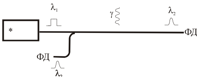
Рис. 2 Принципиальная схема люминесцентного оптоволоконного сенсора
