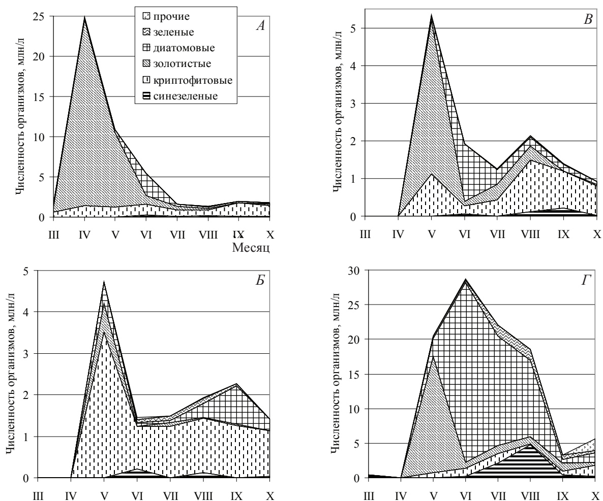
Рис. 3. Сезонная динамика и структурный состав фитопланктонного сообщества ( N_{\text{орг}} , млн орг./л) в 2011 г.: А – оз. Нарочь, Малый плес; Б – оз. Нарочь, Большой плес; В – оз. Мястро; Г – оз. Баторино
