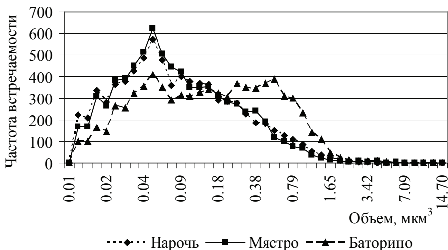
Рис. 6. Частота встречаемости бактериальных клеток разного объема в озерах Нарочь, Мясро и Баторино
