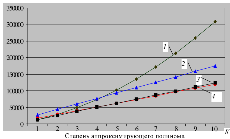
Рис. 1. Количество операций умножения в зависимости от степени приближающего полинома для обычных полиномов МНК (1), Чебышева 1 рода (2), Чебышева 2 рода (3) и Лежандра (4)
