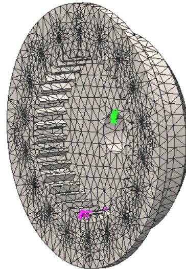
Рис. 3. Параметры сітки (а) та її відображення на твердому тілі (б)
