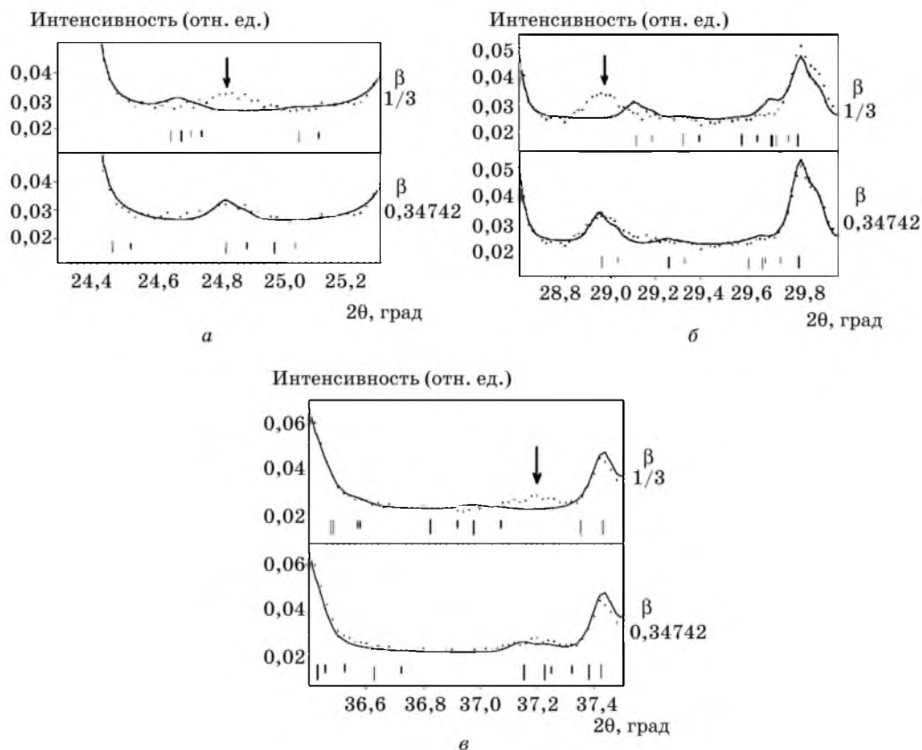
Сопоставление экспериментальной дифракционной кривой (точки) с рассчитанными кривыми (линии) для модуляционных векторов с \beta = 1/3 и \beta = 0,34742 : a — для области 2\theta = 24,4–25,2^\circ ; б — 2\theta = 28,8–29,8^\circ ; в — 2\theta = 36,6–37,4^\circ (вертикальные штрихи показывают положения рефлексов)
