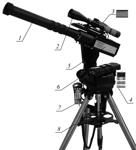
Рис. 1. ССП-600 на поворотной платформе: 1 – бленда с поляридом; 2 – визир оптический; 3 – смартфон для управления ССП-600; 4 – смартфон для управления монтировкой; 5 – спектрополяриметр ССП-600; 6 – аккумулятор; 7 – пульт управления монтировкой; 8 – монтировка
