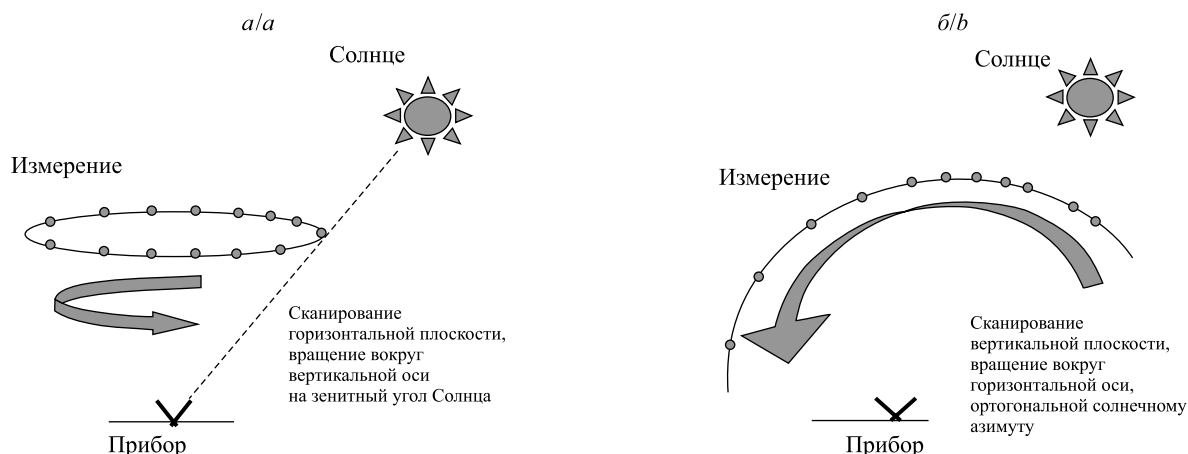
Рис. 5. Схема измерений ССП-600: в альмукантарате Солнца (а); в плоскости солнечного вертикала (б)
