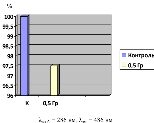
Рисунок 2 – Изменение триптофановой флуоресценции гемоглобина на 10 сутки после острого \gamma -облучения в дозе 0,5 Гр
