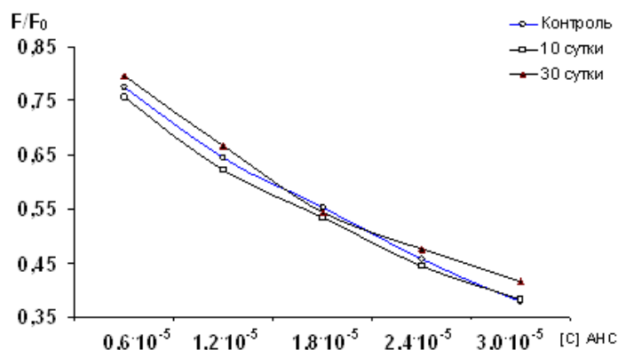
Рисунок 4 – Тушение флуоресценции остатков триптофана гемоглобина при добавлении флуоресцентного зонда АНС к препаратам облучённых животных в дозе 0,5 Гр: F_0 – интенсивность флуоресценции в отсутствие акцептора, F – интенсивность флуоресценции в присутствии акцептора
