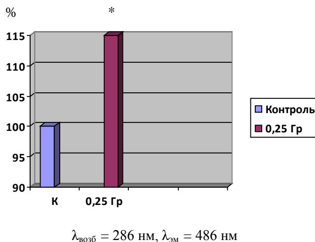
Рисунок 1 – Изменение триптофановой флуоресценции гемоглобина на 10 сутки после острого \gamma -облучения в дозе 0,25 Гр
