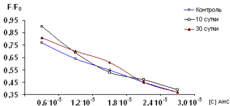
Рисунок 3 – Тушение флуоресценции остатков триптофана гемоглобина при добавлении флуоресцентного зонда АНС к препаратам облучённых животных в дозе 0,25 Гр: F_0 – интенсивность флуоресценции в отсутствие акцептора, F – интенсивность флуоресценции в присутствии акцептора
