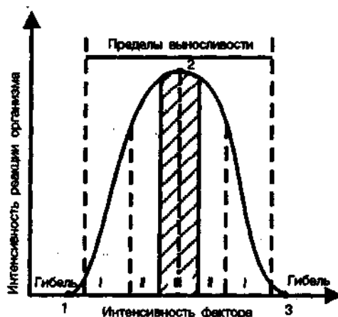
Рис 1. Схема действия экологического фактора на жизнедеятельность организмов: 1, 2, 3 — точки минимума, оптимума и максимума соответственно; I, II, III — зоны пессимума, нормы и оптимума соответственно.
