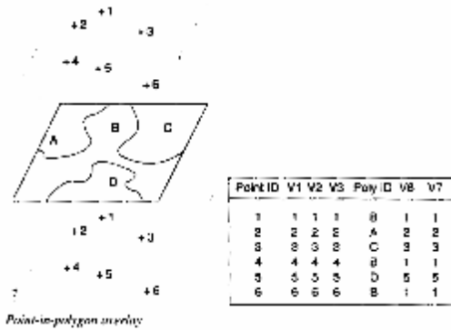
Рис.23. Оверлейная операция пространственного анализа – точка в полигоне
