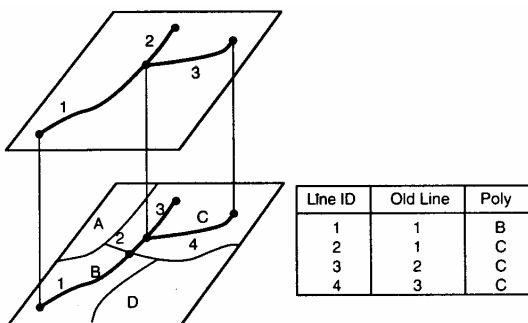
Рис.22. Оверлейная операция пространственного анализа – дуга в полигоне
