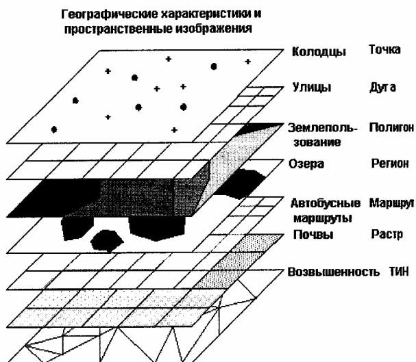
Рис.15. Географическая связка, составленная из разных моделей данных ГИС для определенной местности
