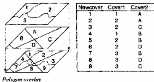
Рис.21. Операция пространственного анализа – полигональный оверлей
