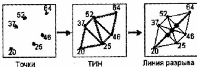
Рис.13. Линии разрыва в TIN модели данных
