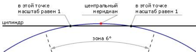
Рис.17. Проекционные преобразования в проекции UTM
