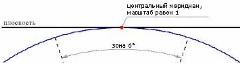
Рис.16. Проекционные преобразования для проекции Гаусса-Крюгера
