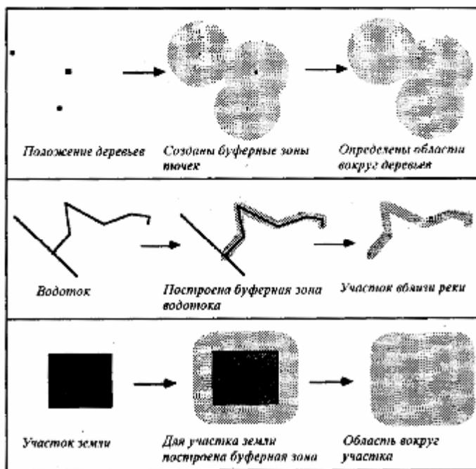
Рис.26. Создание буферных зон вокруг точек, линий или полигонов.
