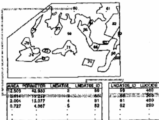
Рис.6. Геореляционная модель данных в ГИС ARC/INFO [1]
