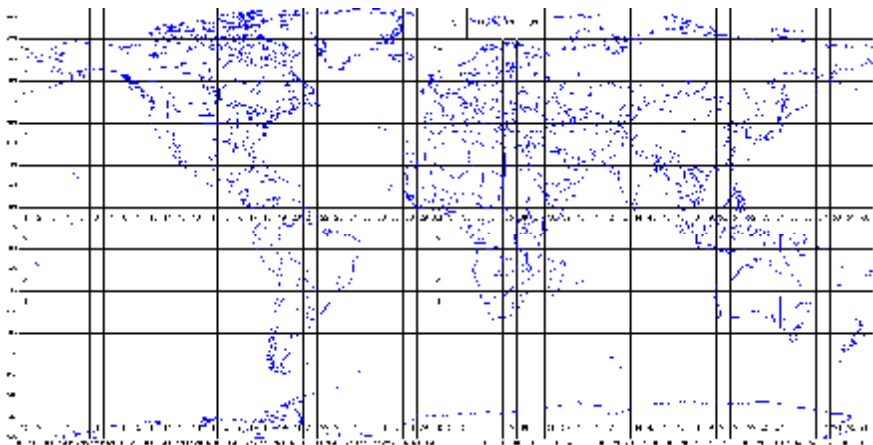
Рис.18. UTM зоны по поверхности земного шара [52]
