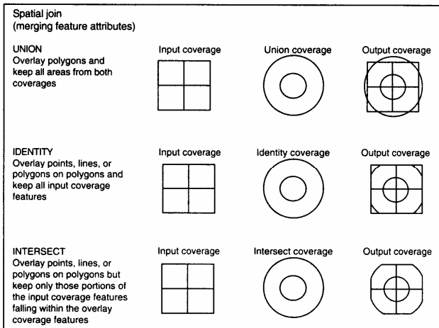
Рис.24. Виды полигональных оверлейных операций в ГИС ARC/INFO
