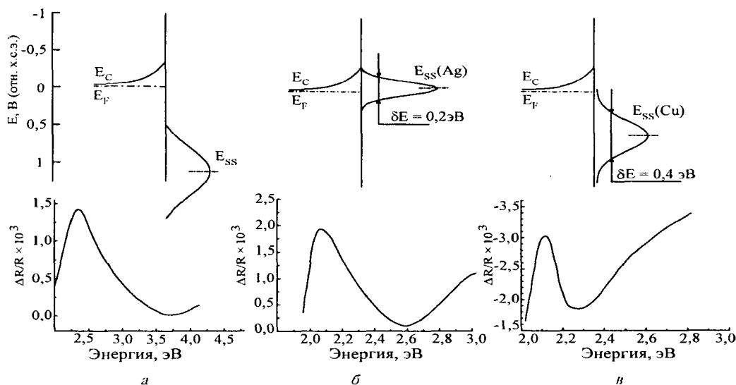
Рис. 1. Спектры электроотражения и энергетические диаграммы контакта полупроводник/электролит для аморфно-кристаллического \text{TiO}_2 : исходного (а); модифицированного осаждением частиц Ag (б); модифицированного осаждением частиц Cu (в). Потенциал электрода: +0,8 В (отн. х. с. э.). Концентрация осажденного металла: \sim 10^{15} \text{ ат. см}^{-2}
