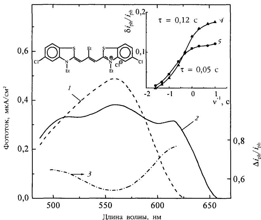
Рис. 3. Спектры фототока для WO_3 -электрода, сенсibilизированного адсорбцией тиокарбонинового красителя в мономолекулярном состоянии (1); частично агрегированного за счет сосаждения с 1,10-декаметилеи-бис-(пиридиний)дибромидом (2, 3). Потенциал электрода: +0,6 В (отн. х. с. э). 3 – спектральное распределение относительного изменения фототока в результате облучения на длине волны 560 нм при потенциале +0,6 В. На врезке приведена частотная зависимость относительного изменения сенсibilизированного фототока для красителя в мономолекулярном (4) и частично-агрегированном (5) состоянии при возбуждении реакции фотоокисления в полосе поглощения мономера (560 нм); потенциал электрода модулировался в диапазоне от +0,5 до -0,2 В
