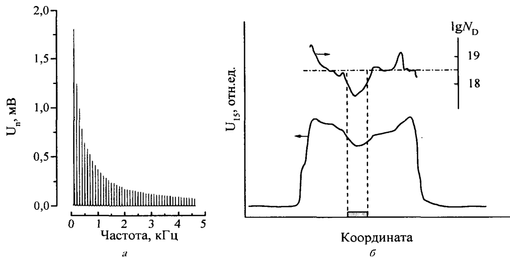
Рис. 2. а – спектр гармоник фотопотенциала аморфно-кристаллического TiO_2 -электрода в условиях облучения импульсным азотным лазером (длительность импульса 10 нс, частота следования импульсов 100 Гц). Потенциал электрода +0,44 В. Электролит: 0,25 М Na_2SO_4 . б – координатные зависимости амплитуды 15-й гармоники фотопотенциала и величины концентрации ионизованных доноров (является функцией dU_n/dE ), полученные при сканировании поверхности аморфно-кристаллического TiO_2 -электрода лазерным лучом. Дефект на электродной поверхности (точка отжига) отмечен штриховкой
